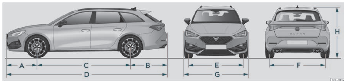
Bild 218 Mått.
