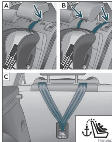
Bild 29 Baksäten: justering och montering enligt Top Tether-bälte
