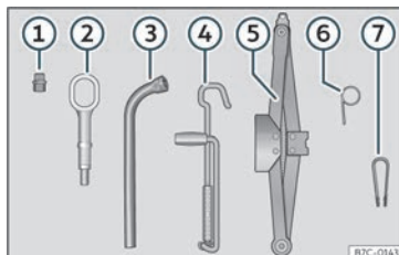
Bild 33 Under golvpanelen i bagageutrymmet: Verktygssats.
