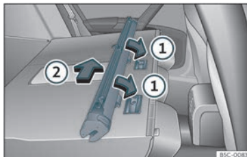
Bild 123 Montering av nätmellanvägg i baksätets ryggstöd.
