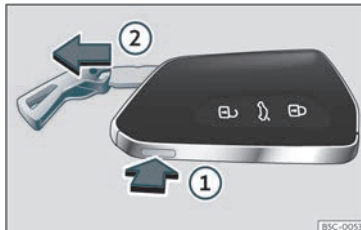
Bild 71 Bilnyckel: ta ut nyckelbladet.
