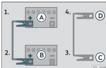
Bild 42 Skiss över anslutning i fordon med startstopp-system.
