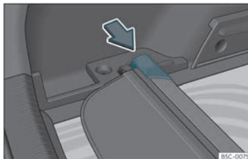
Bild 112 I bagagerummet: I bagageutrymmet: utrymme för att förvara den indragbara hyllan.
