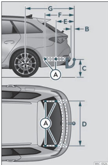
Bild 188 Begränsningar och fästpunkter för eftermontering av en draganordning.
