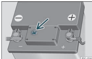
Bild 210 Inspektionsglas ovanpå 12-voltsbatteriet (schematisk framställning).
