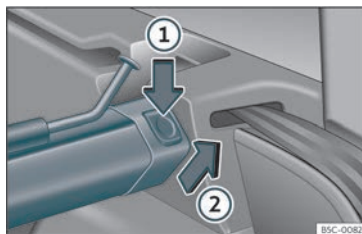
Bild 122 I bagagerummet: Ta bort nätmellanväggen.
