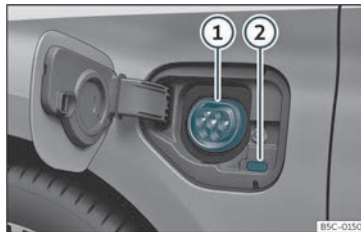
Bild 191 Laddlucka vänster fram bakom batteriet: Laddningsuttag
