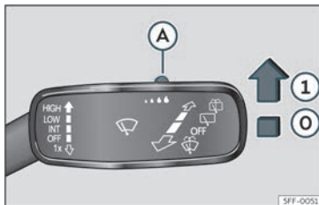
Bild 95 Torkarspak: justering av regnsensor (A).
