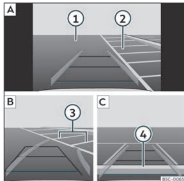
Bild 185 Bild på infotainmentsystemets skärm.: parkering med backassistent.
