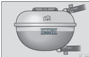
Bild 206 I motorrummet: markering på expansions tanken.
