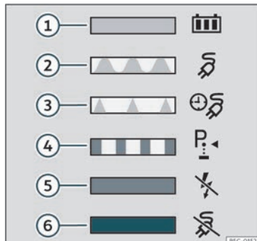
Bild 193 På insidan av luckan till batteriets laddningsuttag: Etikett med information om laddningsdisplayen.
