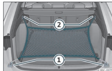
Bild 117 | bagagerummet: fästöglor ① och krokarna ② för att fästa nätpåsen.
